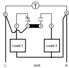
#5 – SPDT
