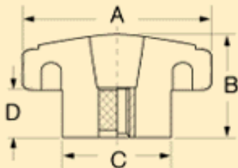
Projecting Stud
