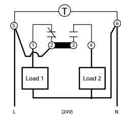
#5 – SPDT
