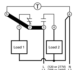
#4 – SPDT
