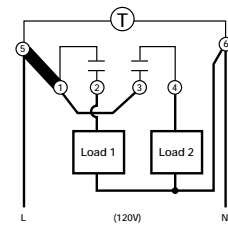
#2 – DPST
