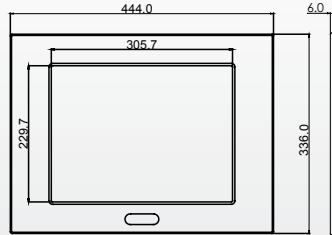
Front Bezel Size
