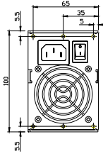
PSA300G(AC-02)
